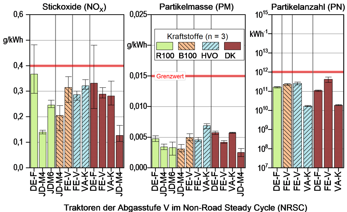
Abbildung 64: Stickoxide (NO x ), Partikelmasse (PM) und Partikelanzahl (PN) von Traktoren der Abgasstufe V mit Rapsölkraftstoff (R100), Biodiesel (B100), hydriertem Pflanzenöl (HVO) und fossilem Dieselkraftstoff (DK)
