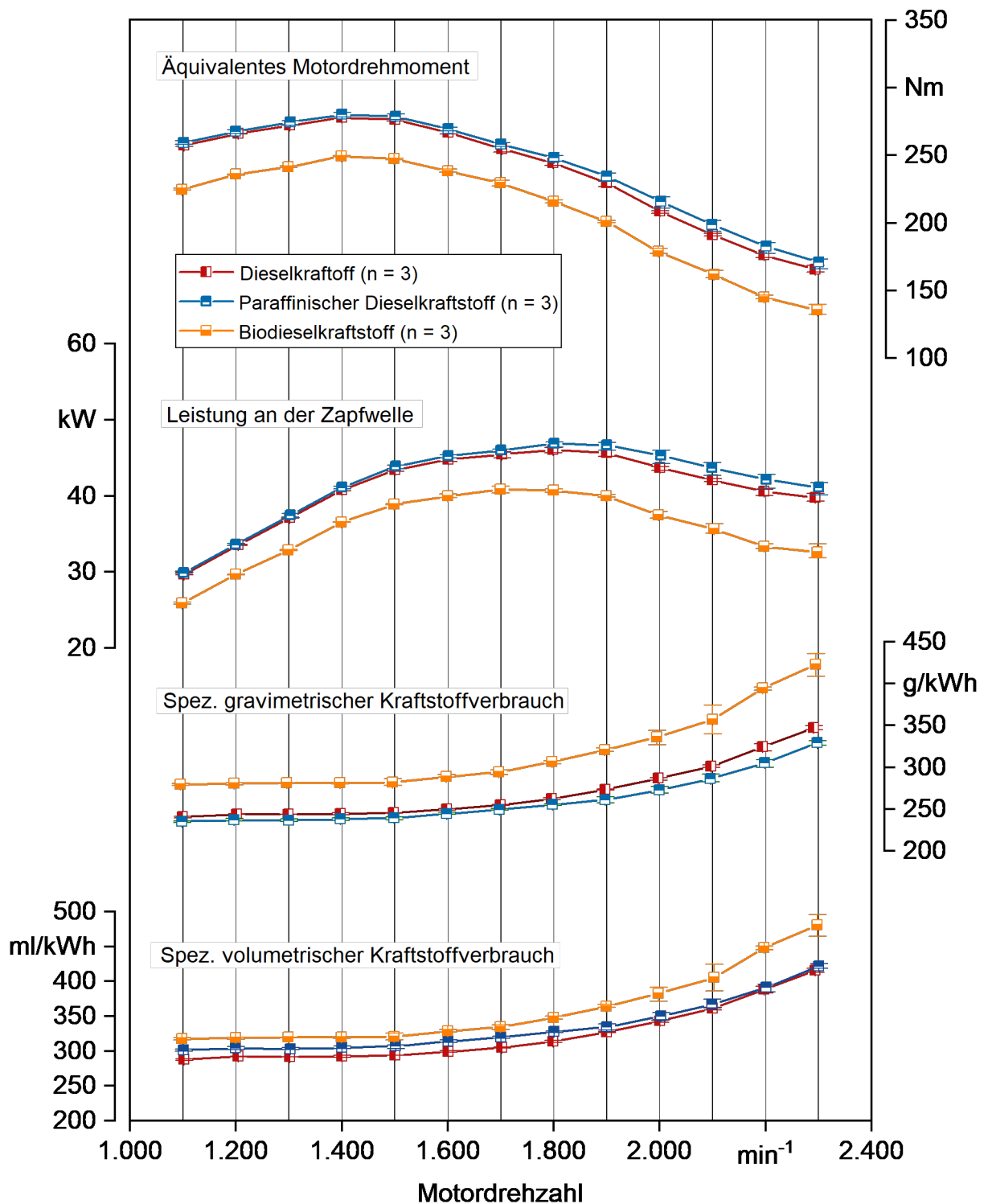
Abbildung 32: Volllastkennlinien des Traktors (ST-S) im Betrieb mit Dieselkraftstoff (DK), paraffinischem Dieselkraftstoff (HVO) und Biodiesel (B100)
