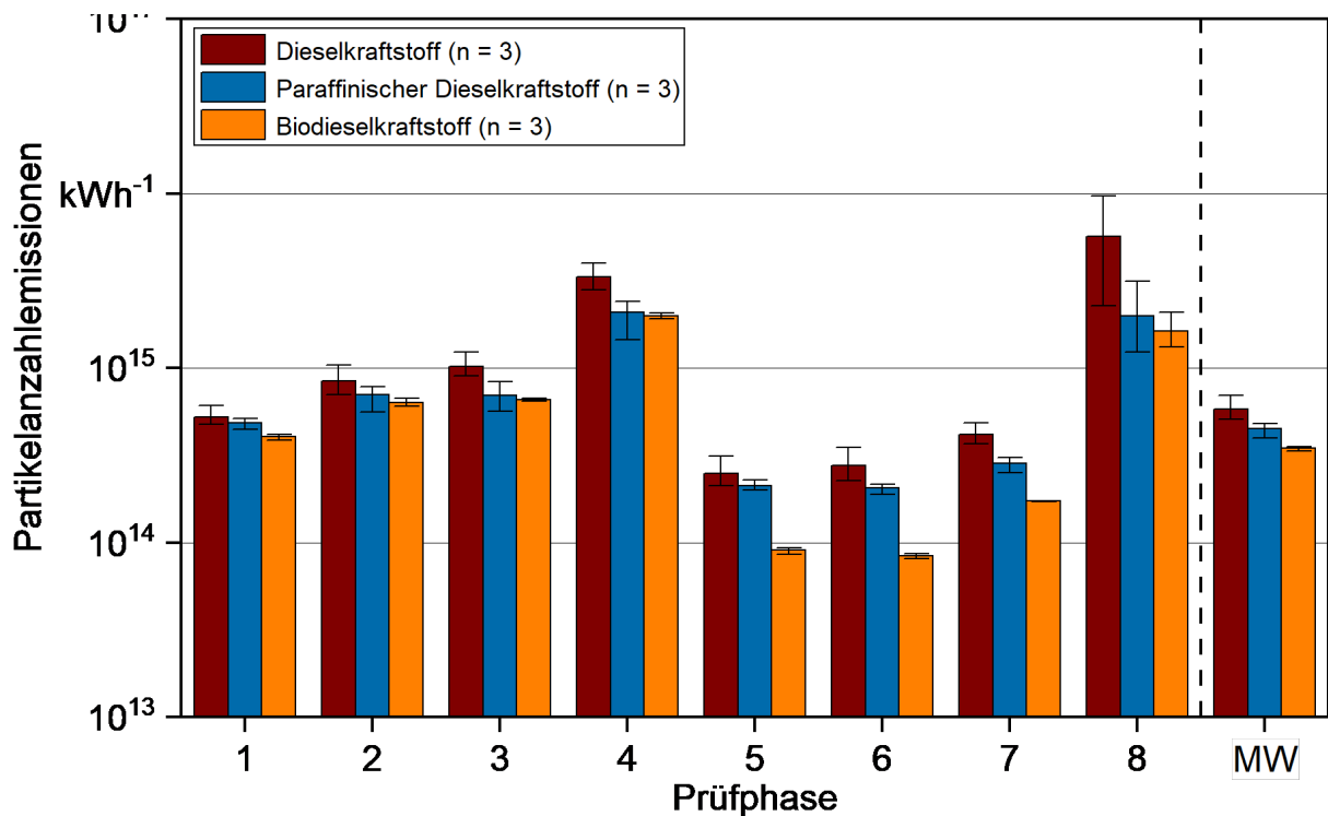
Abbildung 34: Partikelanzahl (Rohemissionen vor Abgasnachbehandlung) des Steyr-Traktors (ST-S) im Betrieb mit Dieseldieselkraftstoff, paraffinischem Dieseldieselkraftstoff (HVO) und Biodieseldieselkraftstoff bei den NRSC-Prüfphasen und als gewichteter Mittelwert (MW)
