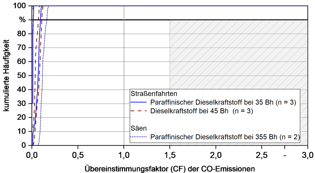
Abbildung 52: Kumulierte Häufigkeit der CO-Emissionen im Verhältnis zum Prüfstandsgrenzwert für die einzelnen Messfahrten des Traktors VA-K mit Dieselmotorkraftstoff und paraffinischem Dieselmotorkraftstoff
