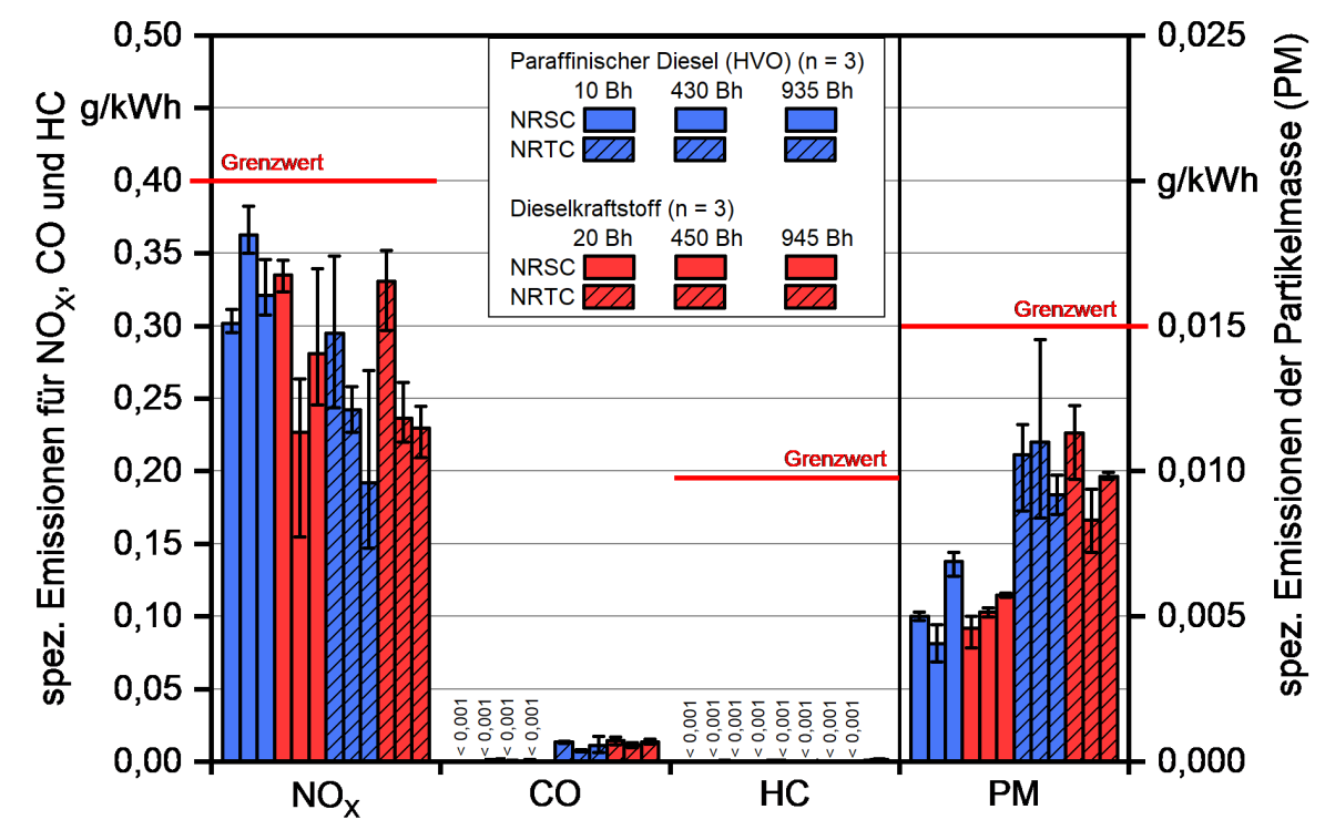
Abbildung 46: NO x -, CO-, HC- und PM-Emissionen des Traktors VA-K beim NRSC und NRTC nach der AGN im Reinabgas mit Dieseldieselkraftstoff und paraffinischem Dieseldieselkraftstoff
