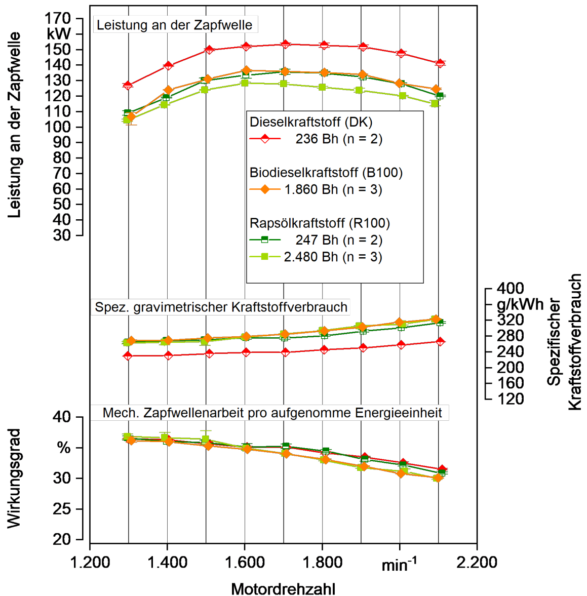
Abbildung 43: Leistung an der Zapfwelle, spezifischer gravimetrischer Kraftstoffverbrauch und Wirkungsgrad an der Zapfwelle des Fendt 724 S4 (FE-S) mit Rapsöl-, Biodiesel- und Dieselskraftstoff
