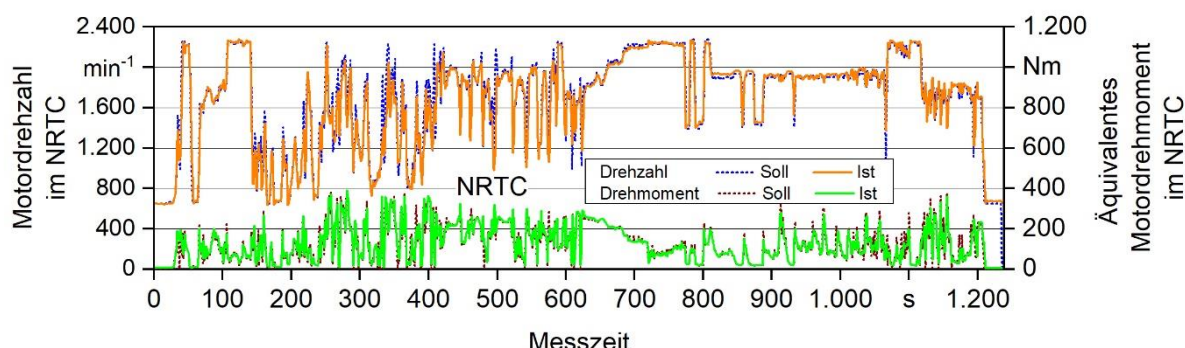
Abbildung 14: Exemplarischer Verlauf der Soll- und Ist-Werte am Traktorenprüfstand des TFZ im NRTC
