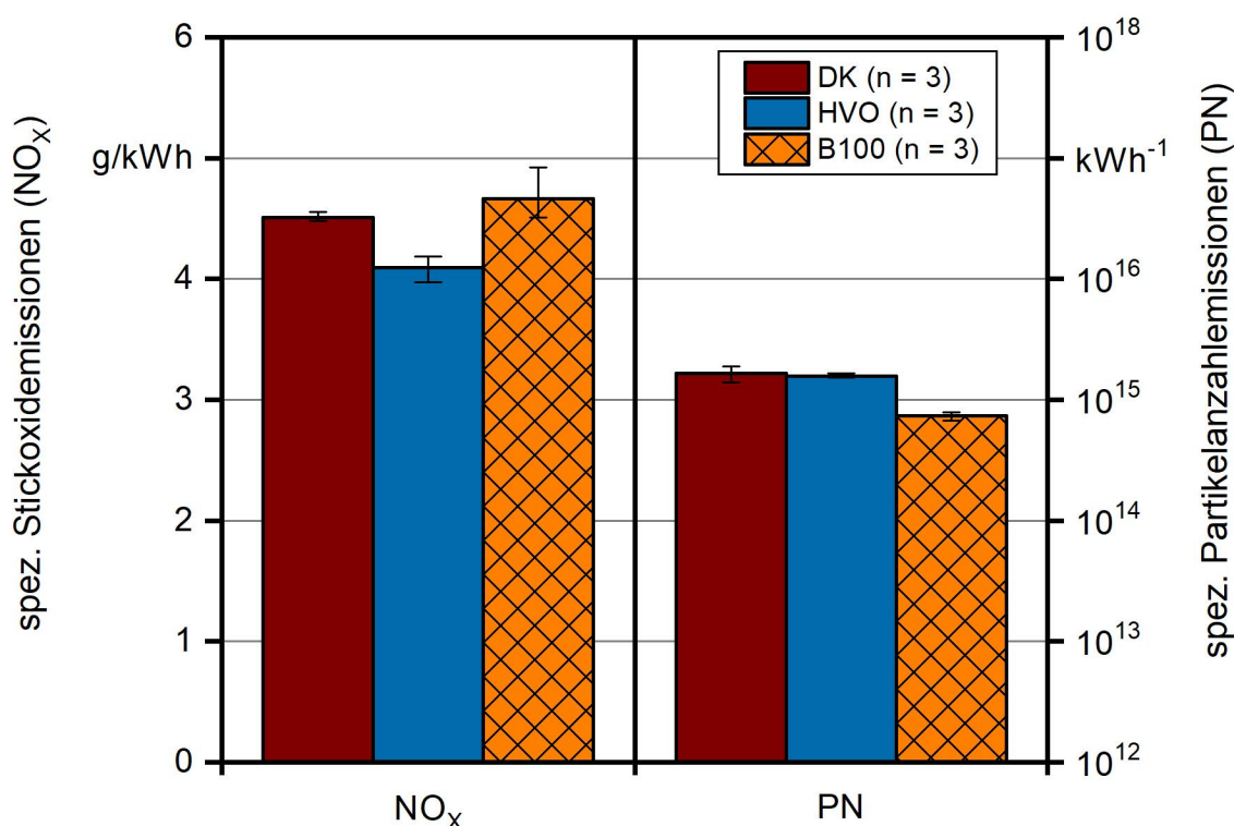
Abbildung 35: Stickstoffoxid- und Partikelanzahlemissionen des Steyr-Traktors (ST-S) im Betrieb mit Dieselkraftstoff (DK), paraffinischem Dieselkraftstoff (HVO) und Biodiesel (B100) im NRTC-Zyklus
