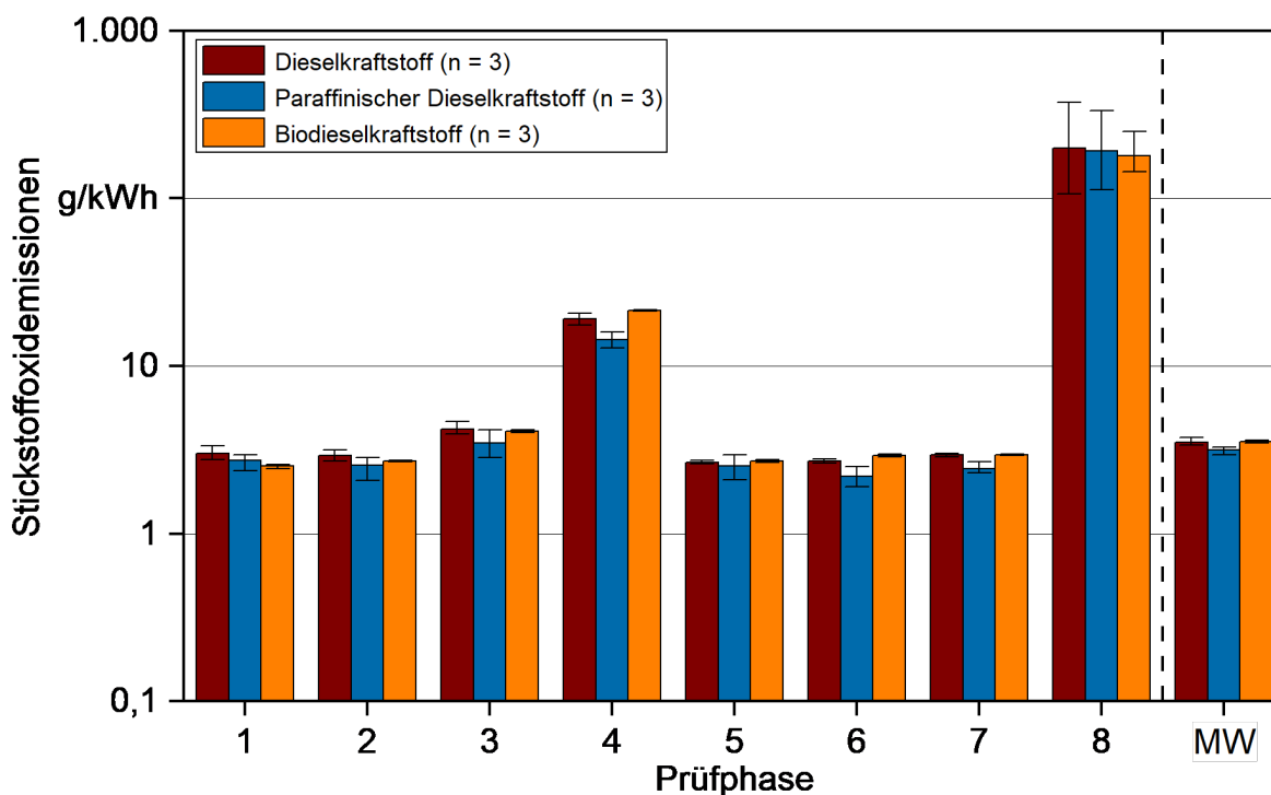
Abbildung 33: Stickstoffoxidemissionen (Rohemissionen vor Abgasnachbehandlung) des Steyr-Traktors (ST-S) im Betrieb mit Dieseldieselkraftstoff (DK), paraffinischem Dieseldieselkraftstoff (HVO) und Biodieseldiesel (B100) bei den NRSC-Prüfphasen und als gewichteter Mittelwert (MW)
