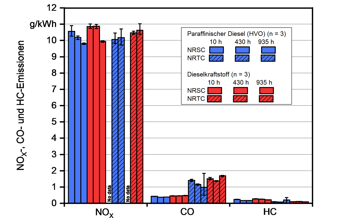
Abbildung 45: NO x -, CO- und HC-Emissionen des Traktors VA-K beim NRSC und NRTC vor der AGN im Rohabgas mit Dieselskraftstoff und paraffinischem Dieselskraftstoff (HVO)
