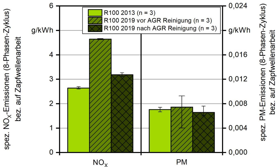
Abbildung 40: Spezifische Stickstoffoxid- (NO x ) und Partikelmasseemissionen (PM) des Traktors John Deere 6210R (JD-P) mit Rapsölkraftstoff (R100) nach der Umrüstung auf Pflanzenölbetrieb im Jahr 2013 sowie vor und nach Reinigung des Abgasrückführsystems (AGR) im März 2019 (Mittelwerte und Schwankungsbreite von je drei Wiederholungsmessungen)
