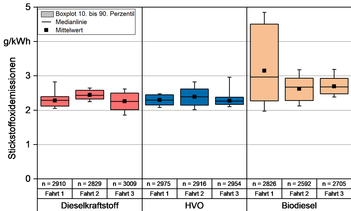
Abbildung 36: Verteilung der spezifischen \text{NO}_x -Emissionen bei Straßenfahrten des Traktors ST-S im Betrieb mit Dieselkraftstoff, paraffinischem Dieselkraftstoff (HVO) und Biodiesel
