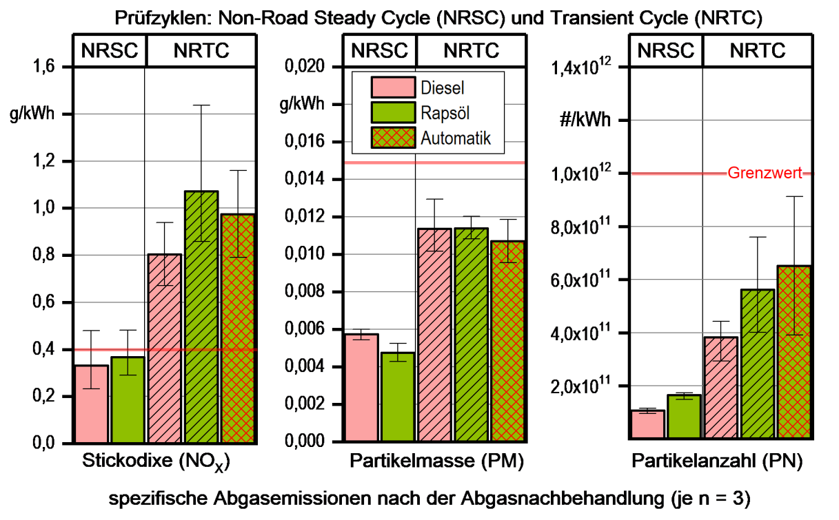
Abbildung 61: NO x -, PM- und PN-Emissionen des Traktors DE-F beim NRSC und NRTC nach der AGN mit Diesel- und Rapsölkraftstoff
