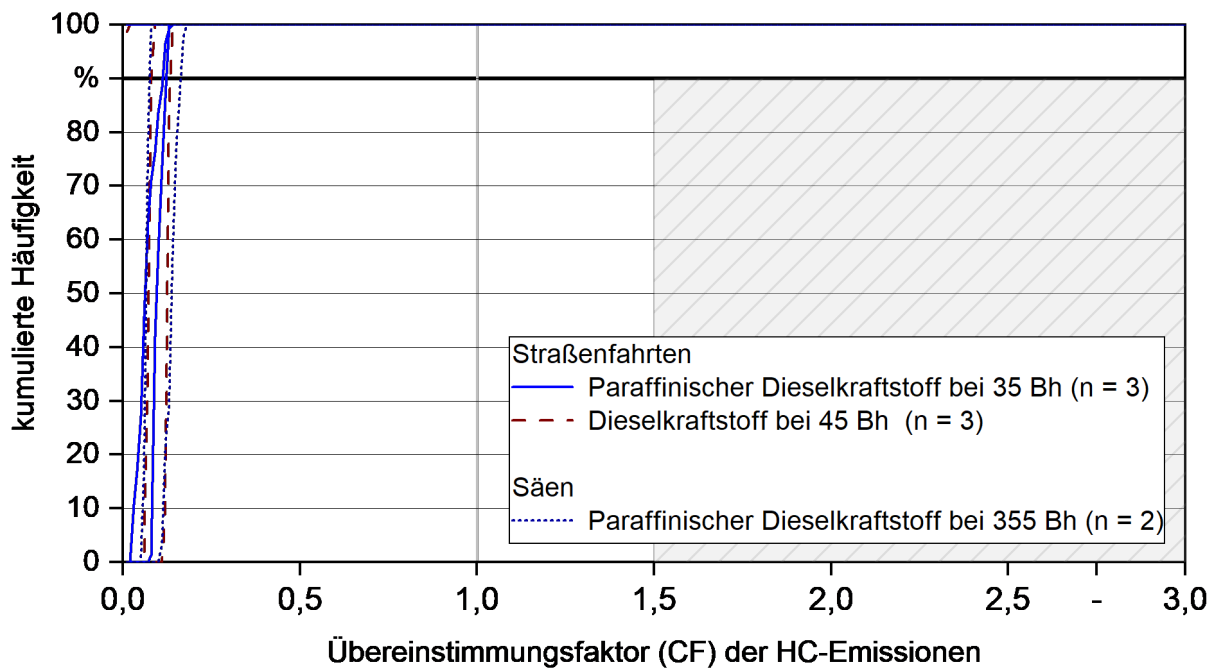
Abbildung 53: Kumulierte Häufigkeit der HC-Emissionen im Verhältnis zum Prüfstandsgrenzwert für die einzelnen Messfahrten des Traktors VA-K mit Dieselmotorkraftstoff und paraffinischem Dieselmotorkraftstoff
