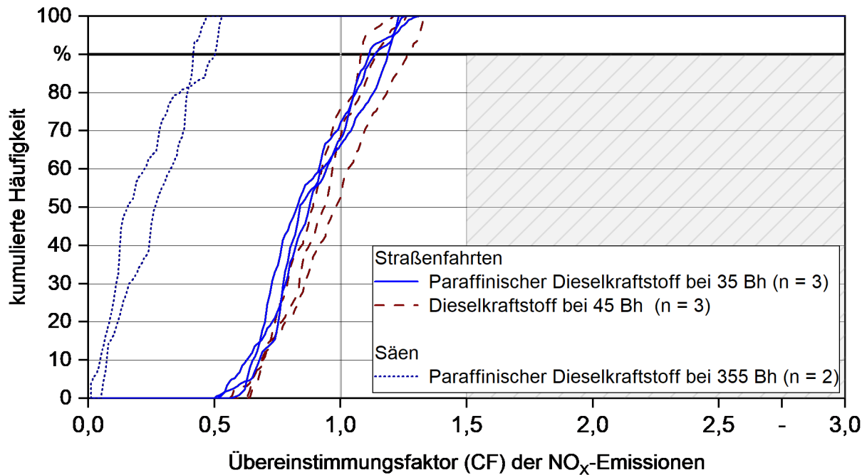
Abbildung 51: Kumulierte Häufigkeit der \text{NO}_x -Emissionen im Verhältnis zum Prüfstandgrenzwert für die einzelnen Messfahrten des Traktors VA-K mit Dieselmotorkraftstoff und paraffinischem Dieselmotorkraftstoff
